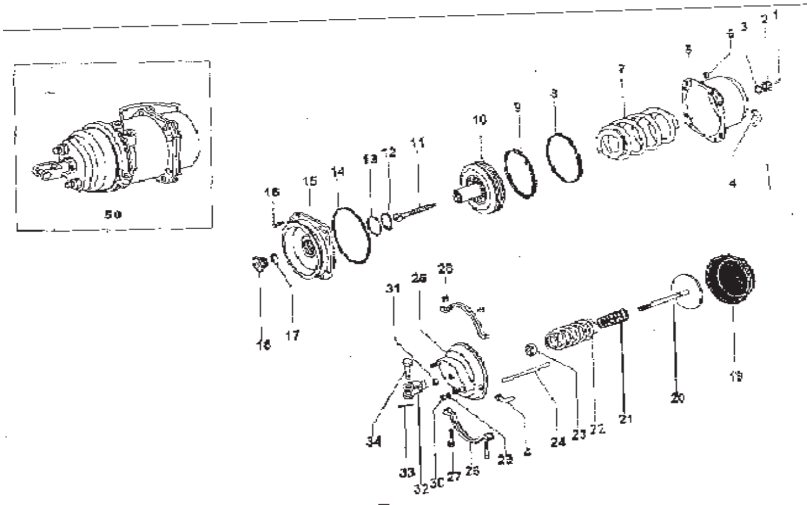
REAR BRAKE ACTUATOR (S-CAM)
